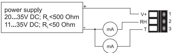
mA...Amperemeter
